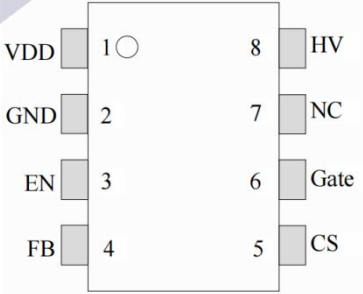
SOP-8俯视图
